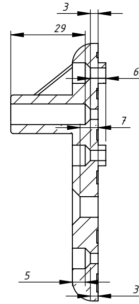
KESIT C-C ÖLÇEK 1 : 1.5
